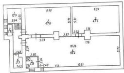
План подвала
