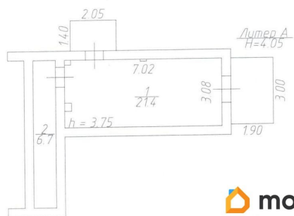
План 1 этажа
