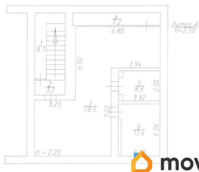
План подвала
