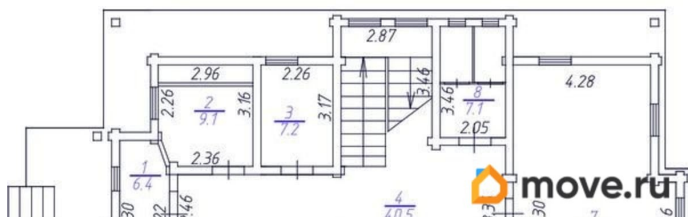
1 Этаж
